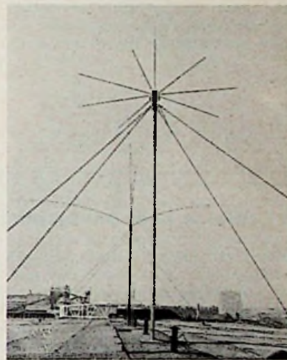
Het actieve drievoudige antennesysteem HE 003. Op de achtergrond een vergelijkbare passieve antenne met antenne elementen die driemaal zo lang zijn.
